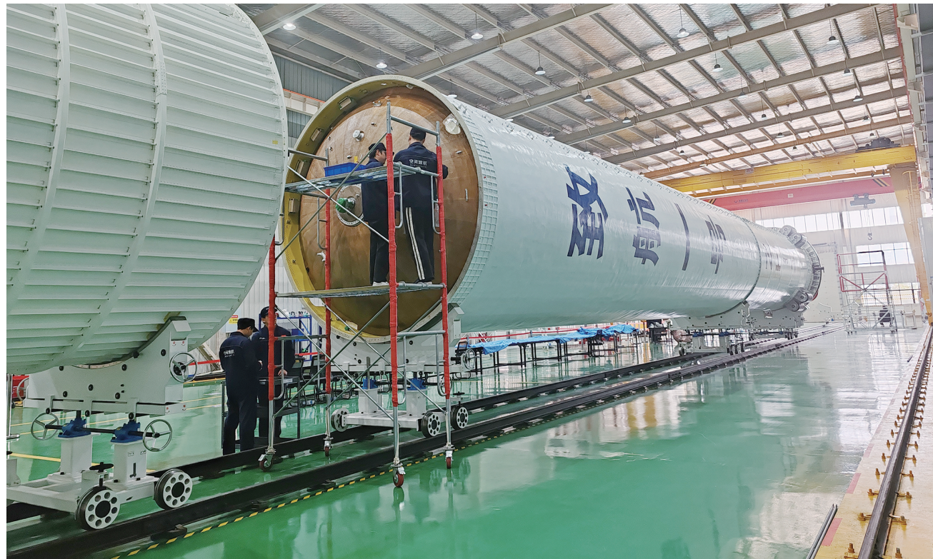
总装车间内,技术人员正在进行精密装配。 全媒体记者 江露露 摄 起。”曹建军说,“从地面改造到空调系统升级,从空气过滤效率到湿度精确控制,我们双方共同努力,硬是在这个临时的厂房里,搭建起一个符合火箭总装条件的空间。” 这个短时间内被“改造”出来的临时厂房,虽不如理想中的宽阔,却成功
